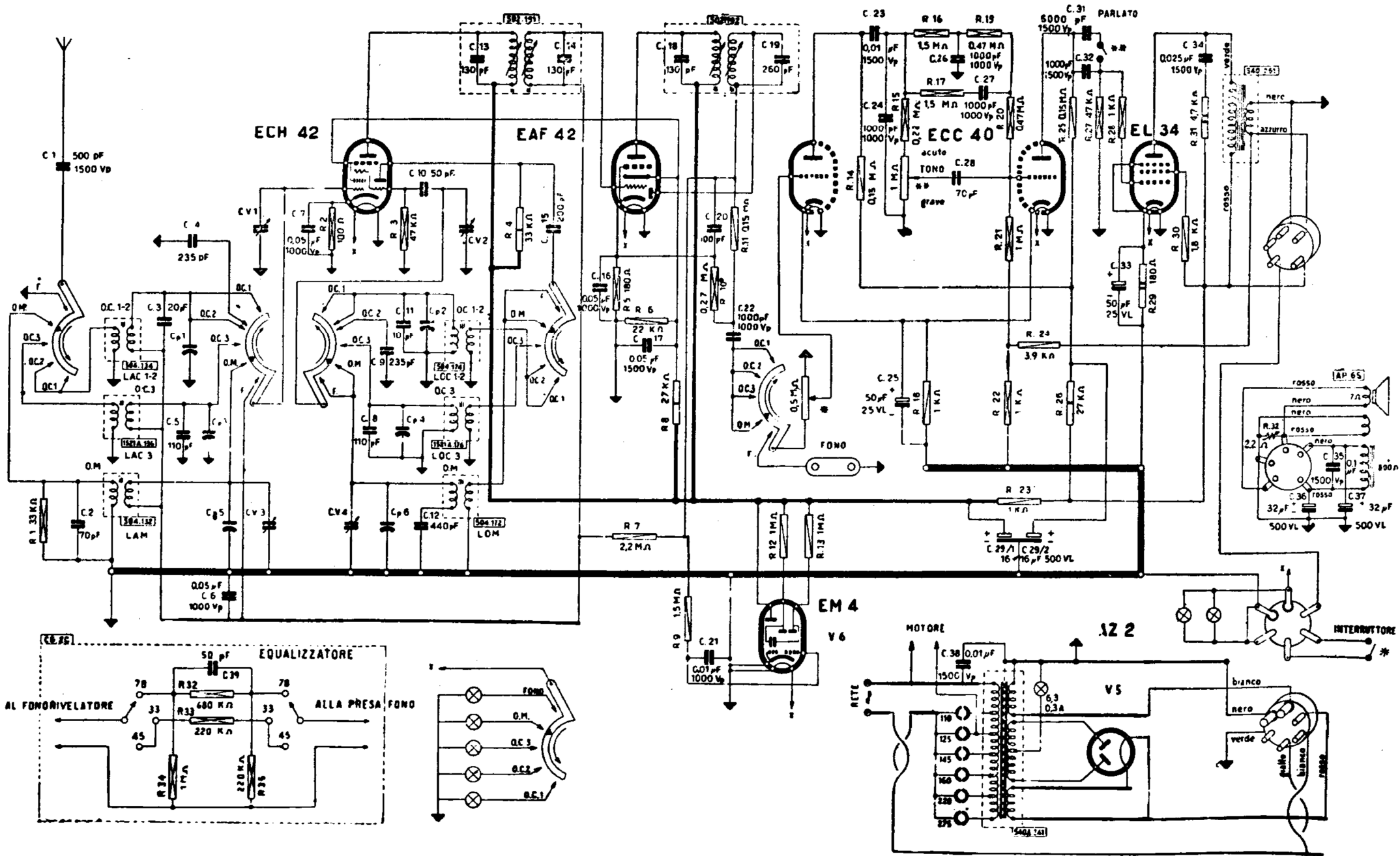
VOCE DEL PADRONE - FONORADIO mod. 545. Onde medie e 2 gamme onde corte, di cui 1 espansa. Media frequenza 465 kc/s. Alimentatore separate. Potenza di uscita 8 watt. Consumo 60 watt.
